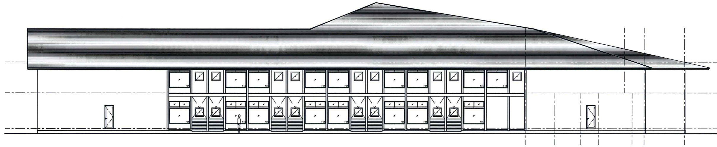
東立面図 S=1/100
