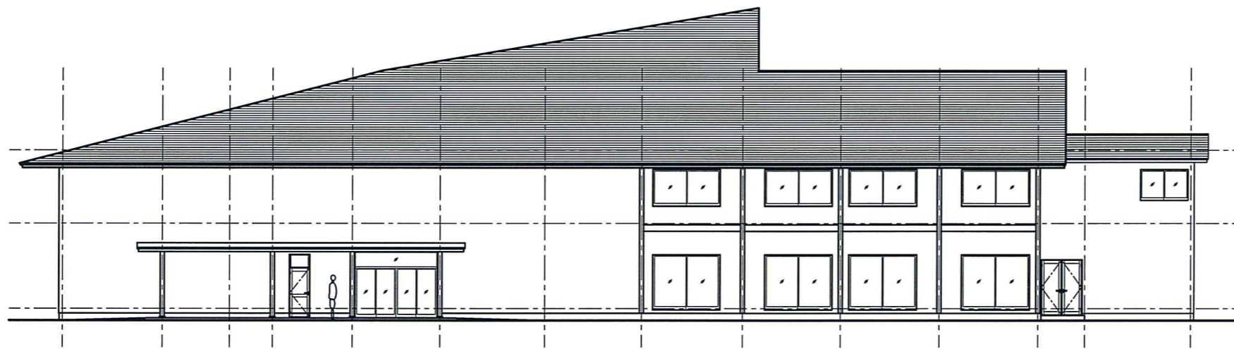
西立面図 S=1/100
